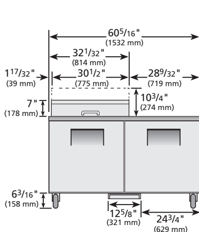
ELEVATION
